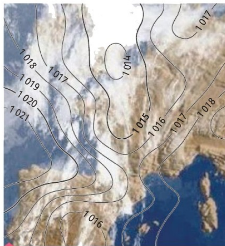
a Images satellitale et carte barométrique (6 juin 2010, 02 h).
