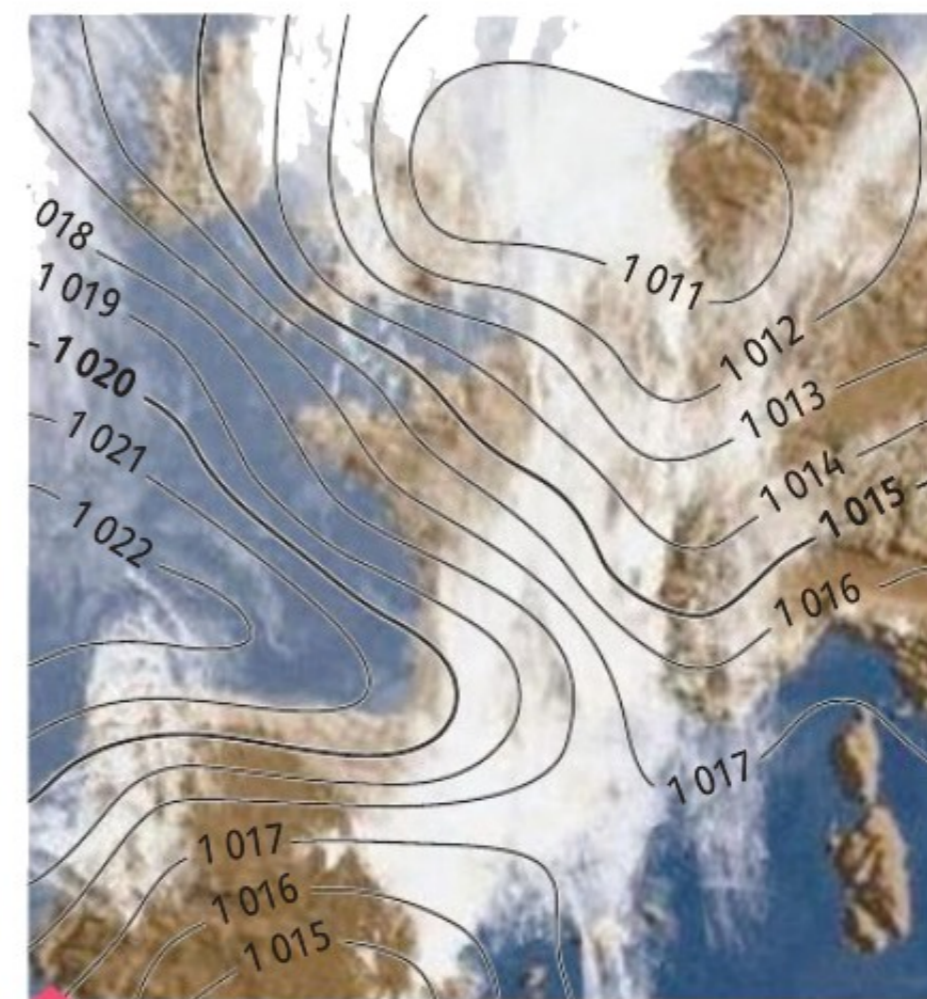
b Images satellitale et carte barométrique (6 juin 2010, 14 h).
